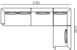
T33ZH-4 3780*2280*700mm 148.8*89.8*27.6"
