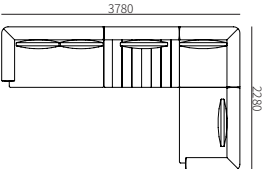
T33ZH-4 3780*2280*700mm 148.8*89.8*27.6"
