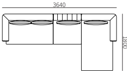
T33ZH-3 3640*1800*700mm 143.3*70.9*27.6"
