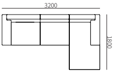
K02ZH-3 3200*1800*760mm 126.0*70.9*29.9"
