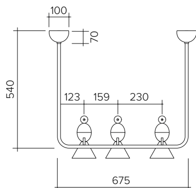
Alouette Pendant 3 Birds 'U' 004OL-C05
