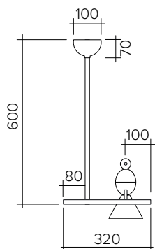
Alouette Pendant 1 Bird 'T' 004OL-C01
