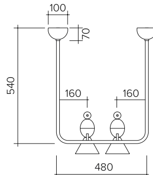
Alouette Pendant 2 Birds 'U' 004OL-C04
