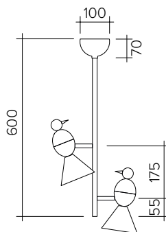
Alouette Pendant 2 Birds 'I' 004OL-C03
